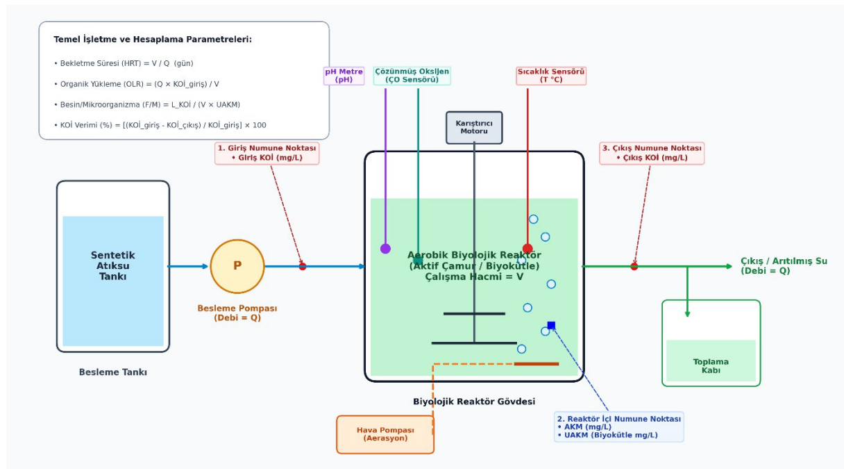
Şekil 3.1. Deney düzeneği.
