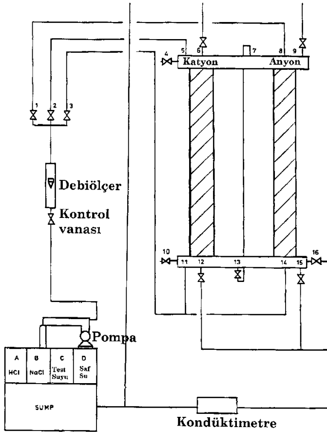
Şekil 9. İyon değişirme deney düzeneğinin vana planı ve şematik durumu
