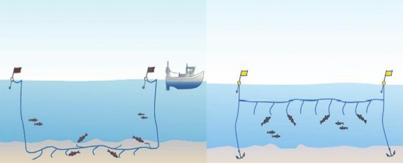
Şekil 4. Dip paraketası (a) ve orta su paraketasının (b) şematik gösterimi
