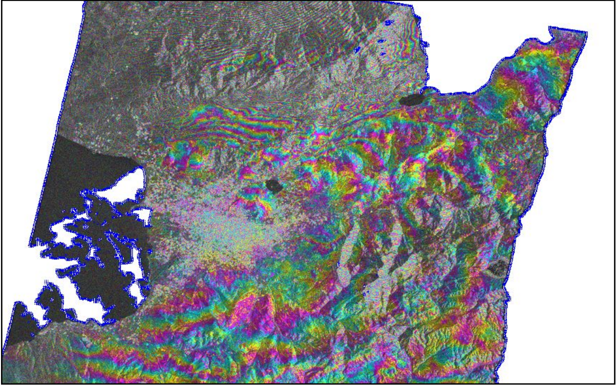
Şekil 5. 23 Ekim 2011 depremi sonrasında COSMO-SkyMed'in verilerinden (10 Ekim - 23 Ekim 2011) Eric, J. Fielding (NASA) tarafından üretilen InSAR görüntüsü.
