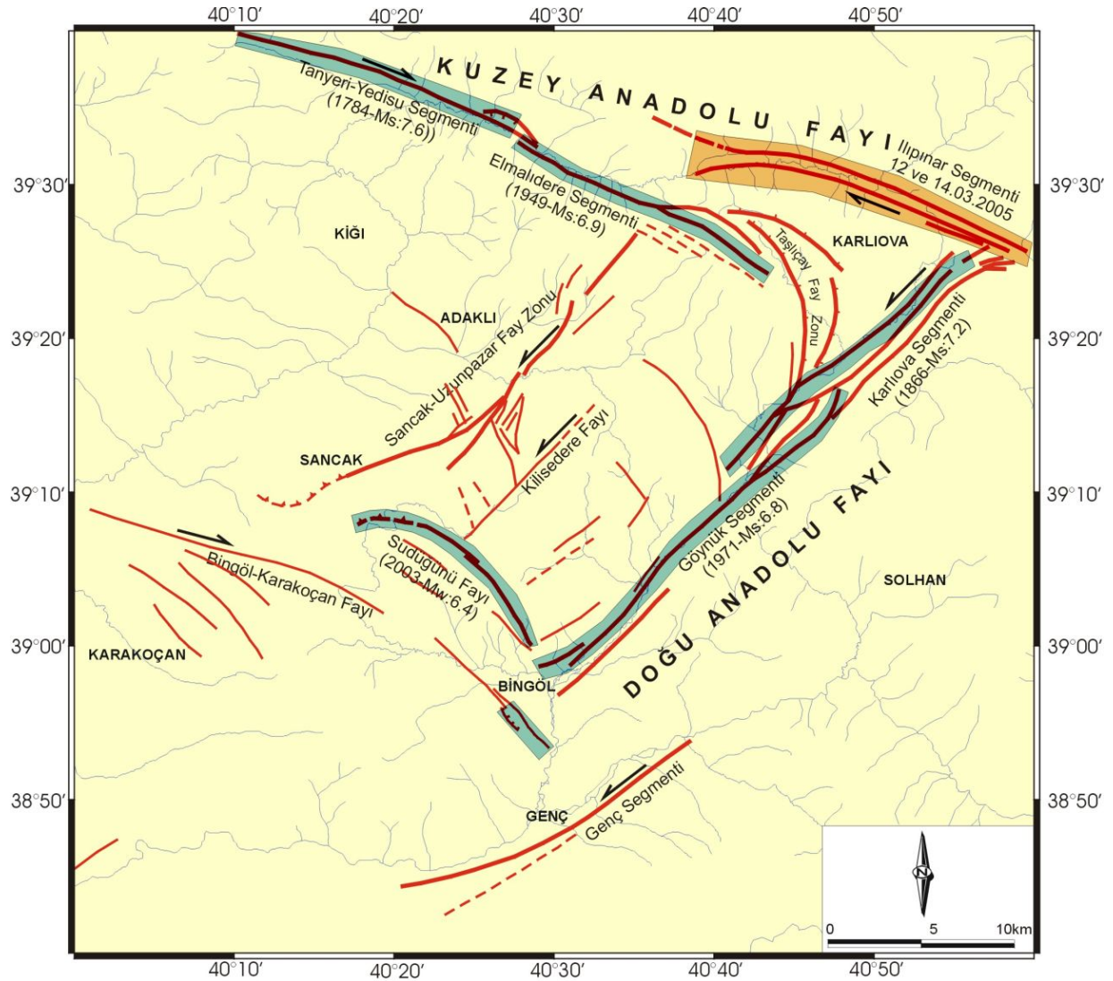
Şekil 4. Karlıova-Bingöl-Kiğı arasındaki diri fay haritası. Sarı bantla gösterilmiş olan KAF'nın Ilıpınar segmenti olasılıkla 12 ve 14 Mart 2005 Karlıova depremlerine kaynaklık etmiştir. Mavi bantla gösterilmiş faylar ise 1784-Günümüz arasında yıkıcı deprem üretmiş fayları gösterir. Bantlanmamış olanlar ise bölgede deprem potansiyeli yüksek olan fay zonlarını gösterir.
